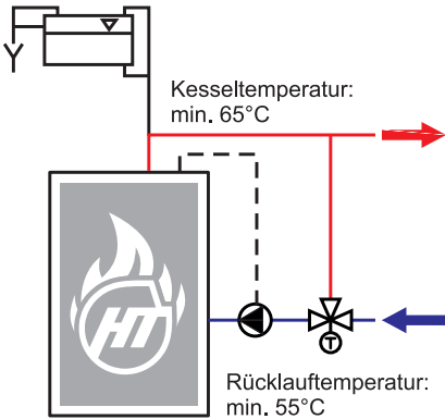
Rücklaufschutz mit Thermostatventilen
